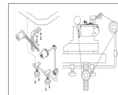
■ RT-1 ゴム張り装置 (手動式) RX-PHK Elastic expander device ( manual operation ) RX-PHK EXPANDIDOR DE ELASTICO RX-PHK 松紧带撑开装置
