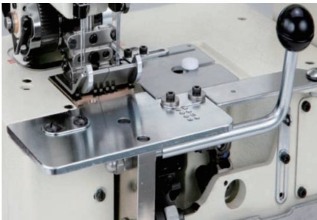
■ TB ターンダウンホルダーブラケット (*1508SPF,1509SPFは標準装備) TURN DOWN FOLDER BRACKET (*This is standard equipment for 1508SPF,1509SPF) EQUIPAMENTO ESTANDAR (PARA 1508SPF, 1509SPF) 拉开式面板 (1508SPF, 1509SPF 标准装备)
